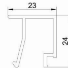
زهوار ۲ جداره ترمال Double rickety Code : 21351 weight : 0.3 kg/m
