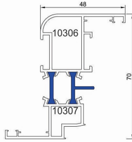
پروفیل لنگه Vent profile Code : 10306-10307 weight : 1.38 kg/m
