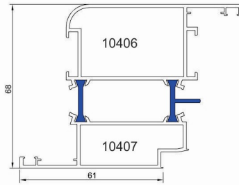
لنگه درب Door vent profile Code : 10406-10407 weight : 1.8 kg/m
