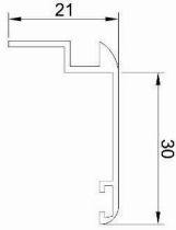
روکوب ۳۰ Suppressed the binding Code : 10022 weight : 0.22 kg/m
