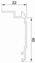
روکوب ۴۰ Suppressed the binding Code : 10025 weight : 0.26 kg/m
