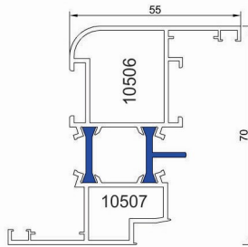
پروفیل لنگه Vent profile Code : 10506-10507 weight : 1.49 kg/m
