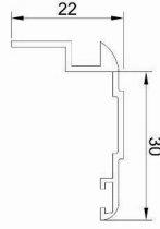
روکوب ۳۰ Suppressed the binding Code : 10023 weight : 0.23 kg/m
