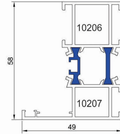
پروفیل فریم Frame profile Code : 10206-10207 weight : 1.2 kg/m
