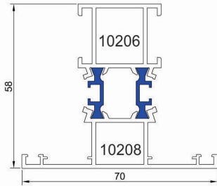
پروفیل سپری T profile Code : 10206-10208 weight : 1.33 kg/m
