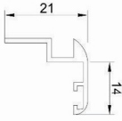
روکوب ۱۴ Suppressed the binding Code : 10021 weight : 0.2 kg/m
