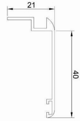
روکوب ۴۰ Suppressed the binding Code : 10024 weight : 0.25 kg/m
