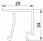
زهوار ۲ جداره ترمال Double rickety Code : 21352 weight : 0.31 kg/m
